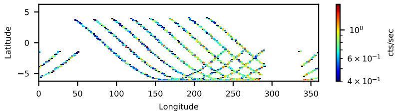
60001041002: 3 to 120 keV
