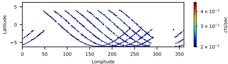
60001041002: 3 to 10 keV
