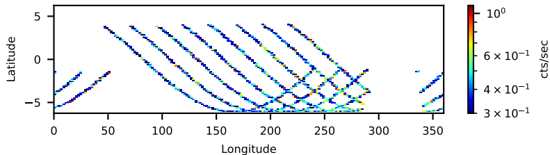
60001041002: 30 to 120 keV
