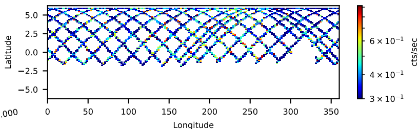
50701001002: 30 to 120 keV
