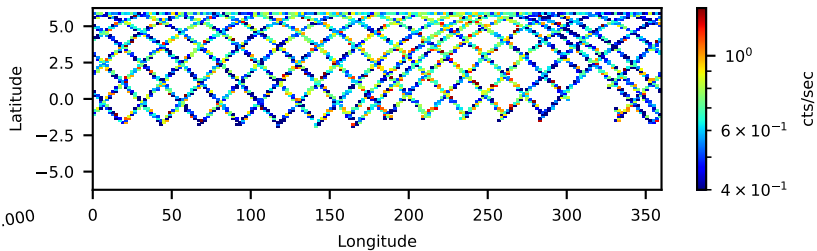
50701001002: 3 to 10 keV
