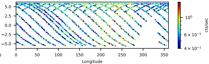
50460004002: 3 to 10 keV
