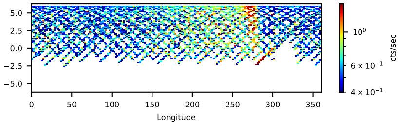
50310003001: 3 to 10 keV
