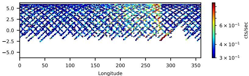
50310003001: 30 to 120 keV
