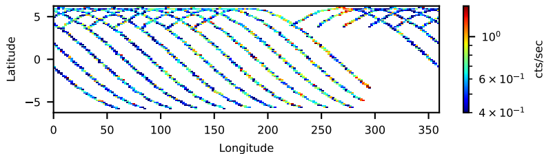
50110002006: 3 to 120 keV
