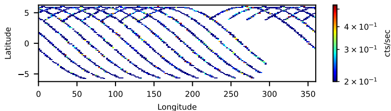
50110002006: 3 to 10 keV
