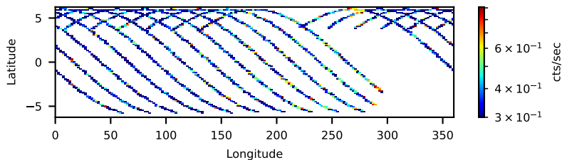
50110002006: 30 to 120 keV
