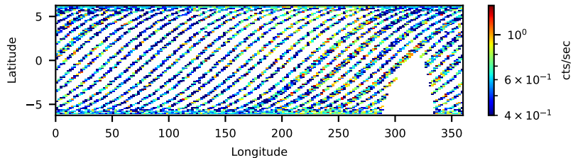
50026003002: 3 to 120 keV
