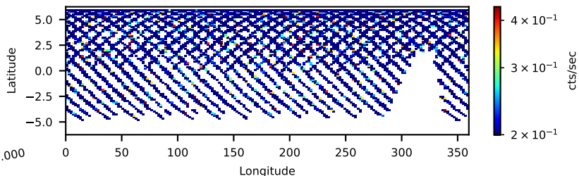
50002031004: 30 to 120 keV
