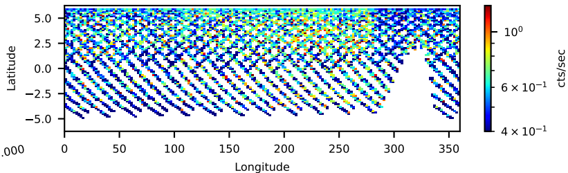
50002031004: 3 to 10 keV
