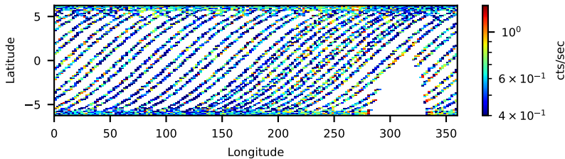
40801006002: 3 to 120 keV
