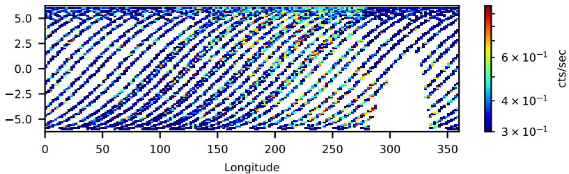
40701008001: 30 to 120 keV
