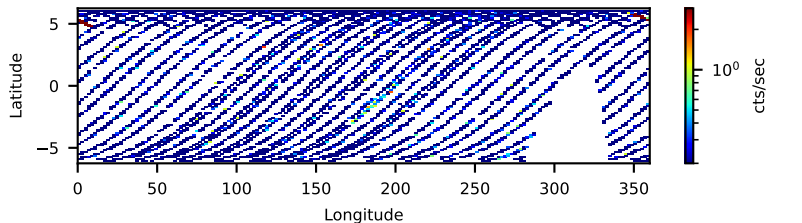
40701008001: 3 to 10 keV
