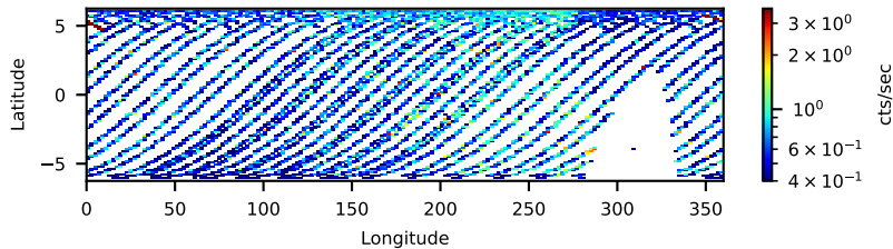
40701008001: 3 to 120 keV
