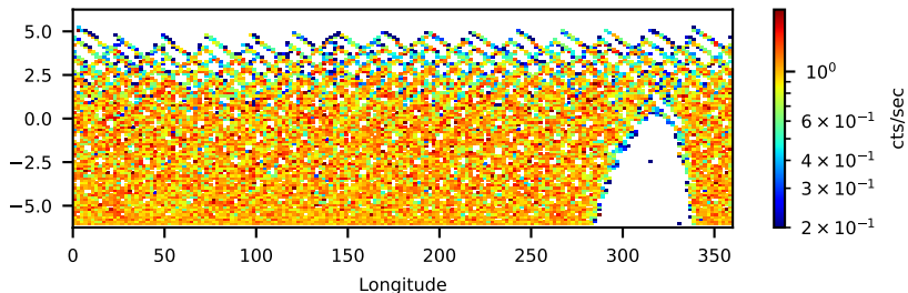
40020001004: 30 to 120 keV
