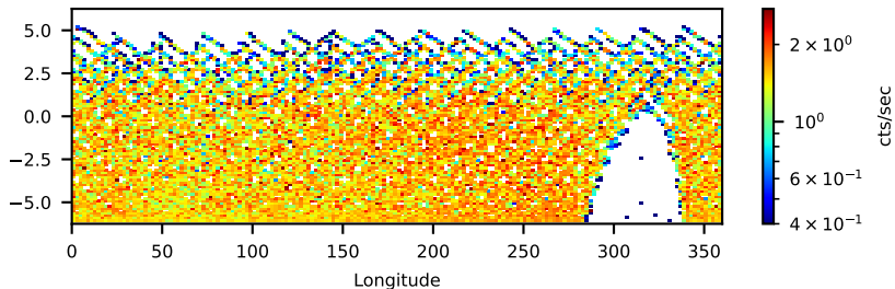
40020001004: 3 to 10 keV
