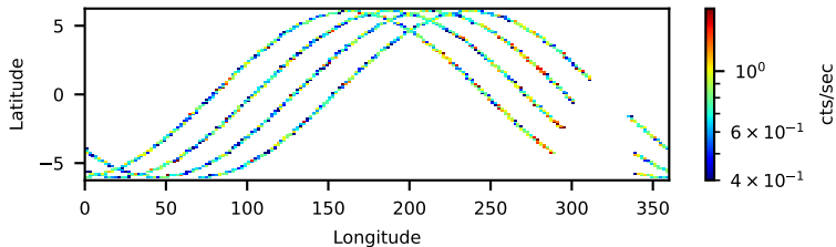
40001014012: 3 to 120 keV
