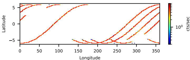
31102015004: 3 to 10 keV
