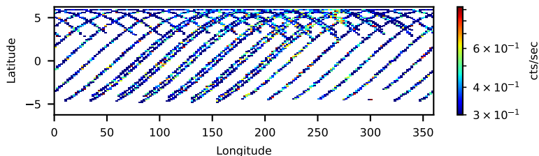
31101025004: 30 to 120 keV
