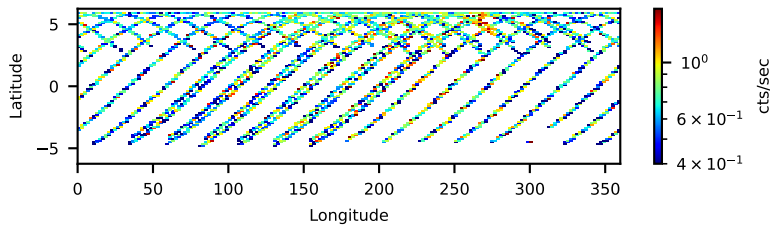
31101025004: 3 to 120 keV
