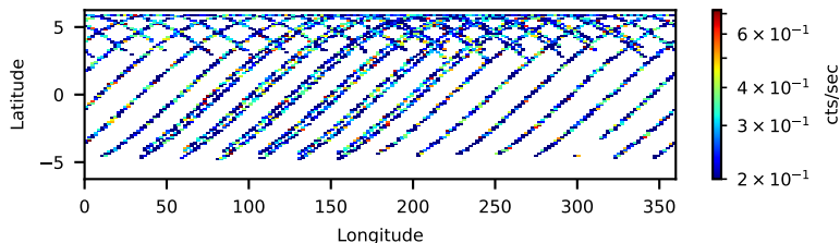
31101025004: 3 to 10 keV
