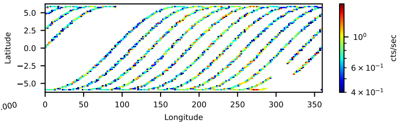
31002008006: 3 to 10 keV
