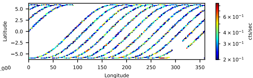
31002008006: 30 to 120 keV
