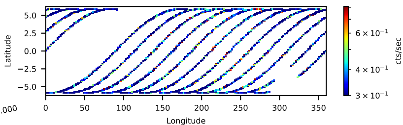
31002008006: 30 to 120 keV
