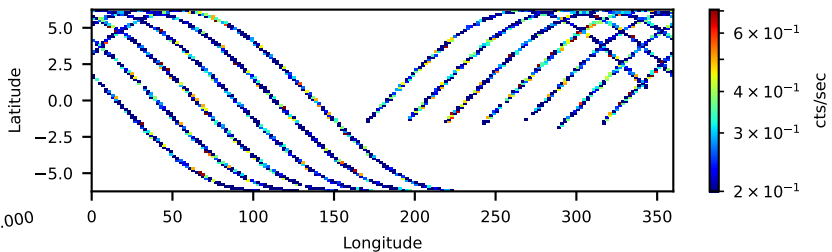
31002003008: 30 to 120 keV
