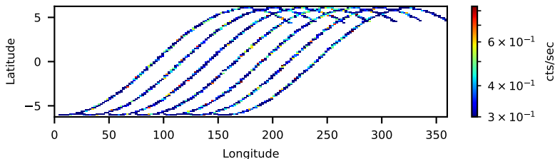
31002003004: 30 to 120 keV
