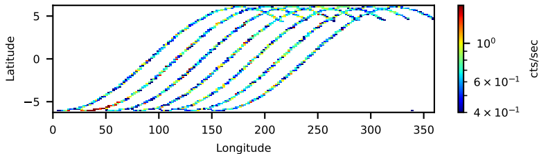
31002003004: 3 to 120 keV
