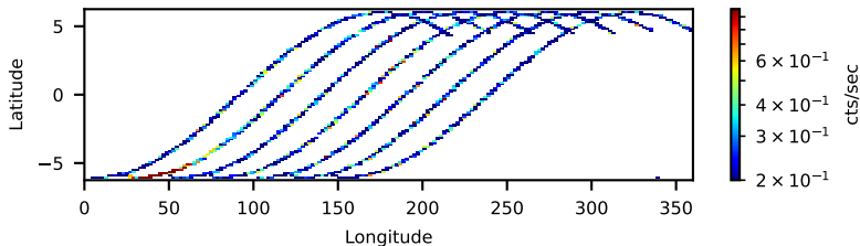
31002003004: 3 to 10 keV
