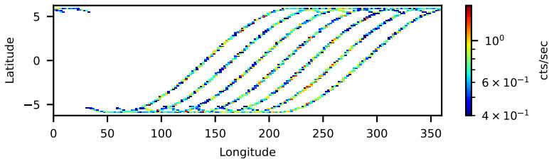
31002003002: 3 to 120 keV
