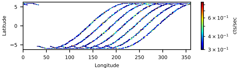
31002003002: 30 to 120 keV
