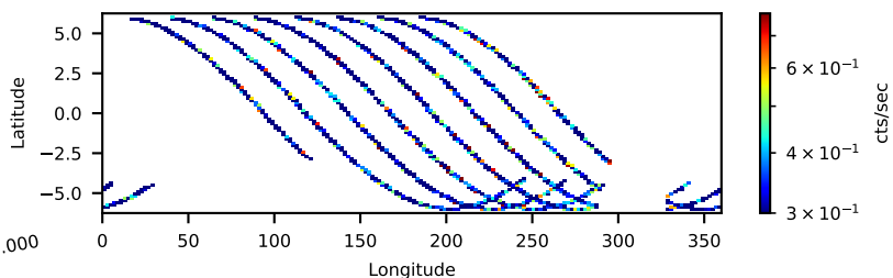
31002002012: 30 to 120 keV
