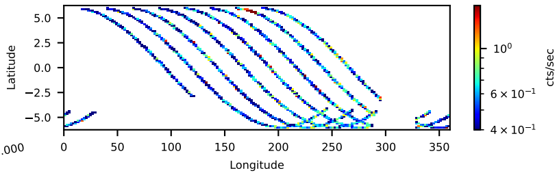
31002002012: 3 to 10 keV
