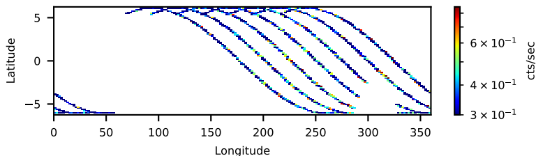
31002002004: 30 to 120 keV
