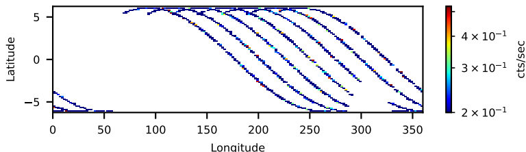
31002002004: 3 to 10 keV
