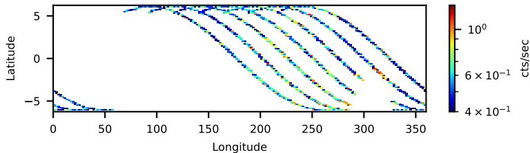
31002002004: 3 to 120 keV
