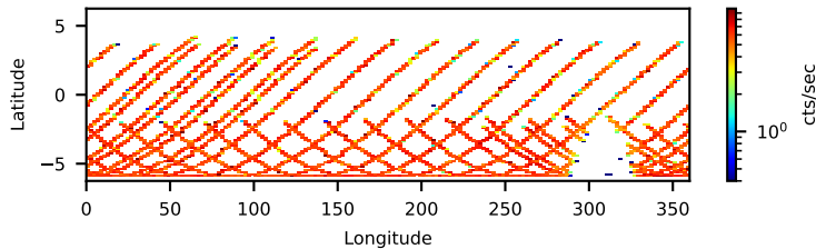
31001012002: 3 to 120 keV
