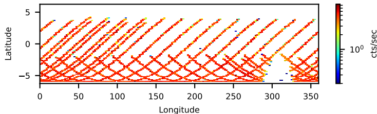
31001012002: 3 to 10 keV
