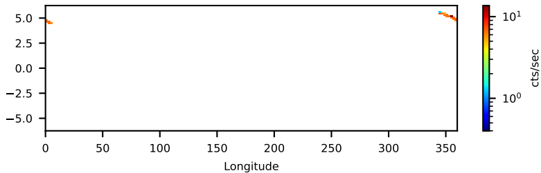
30902026005: 3 to 10 keV
