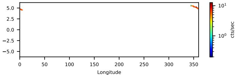
30902026005: 30 to 120 keV
