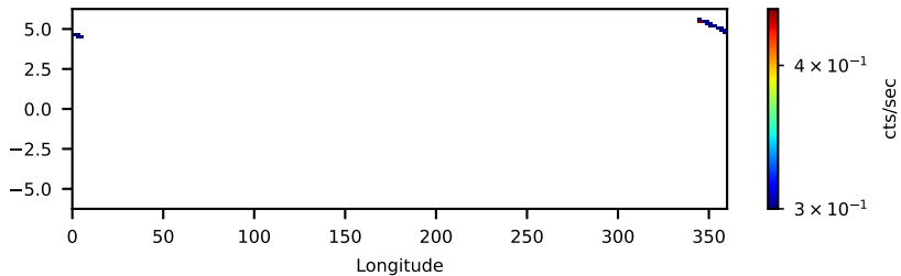
30902026005: 30 to 120 keV
