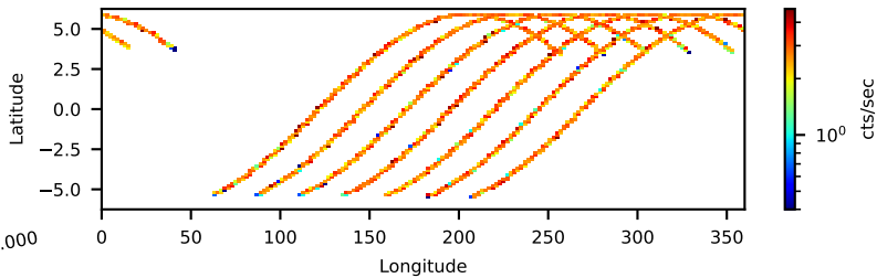
30902013006: 3 to 10 keV
