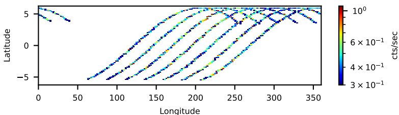
30902013006: 30 to 120 keV
