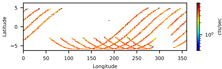
30801024006: 3 to 120 keV
