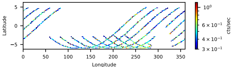
30801024006: 30 to 120 keV
