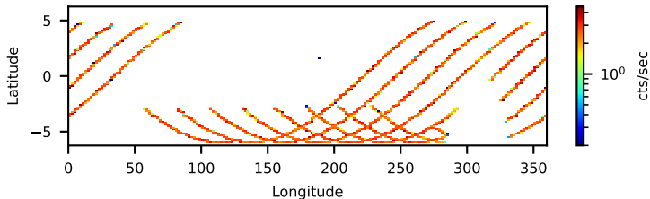
30801024006: 3 to 10 keV
