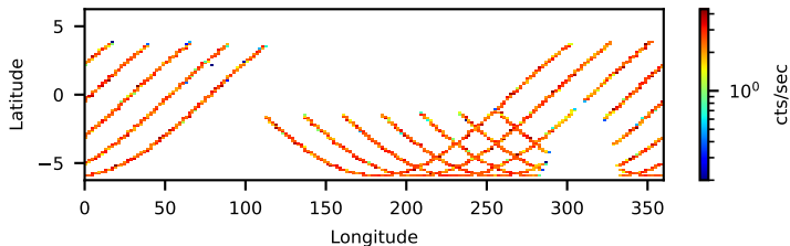
30801024004: 3 to 10 keV
