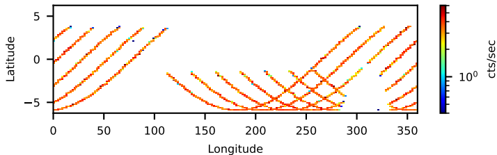
30801024004: 3 to 120 keV
