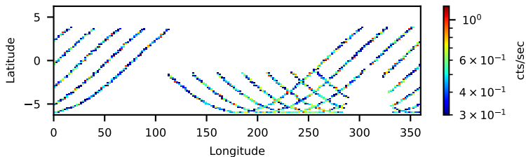
30801024004: 30 to 120 keV
