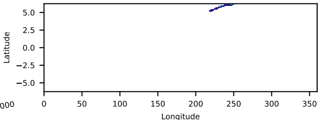
30801023001: 30 to 120 keV
