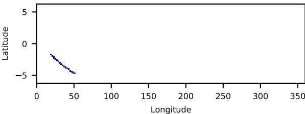
30702018009: 30 to 120 keV
