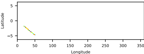
30702018009: 3 to 10 keV
