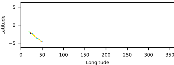
30702018009: 3 to 120 keV
