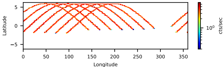
30702017006: 3 to 10 keV
