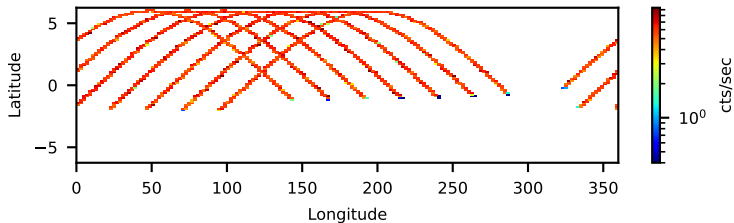
30702017006: 3 to 120 keV
