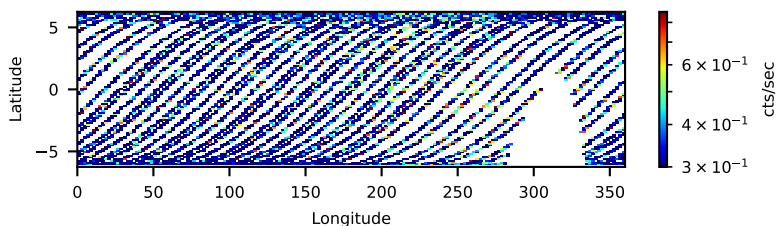
30702012004: 30 to 120 keV
