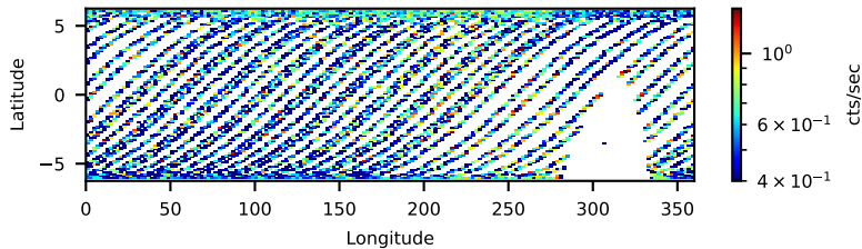
30702012004: 3 to 120 keV
