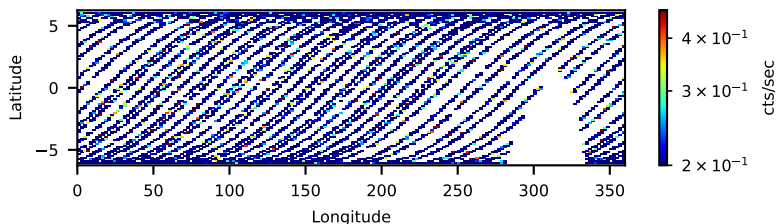
30702012004: 3 to 10 keV
