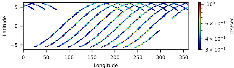
Longitude
