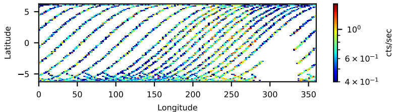
30460019002: 3 to 120 keV
