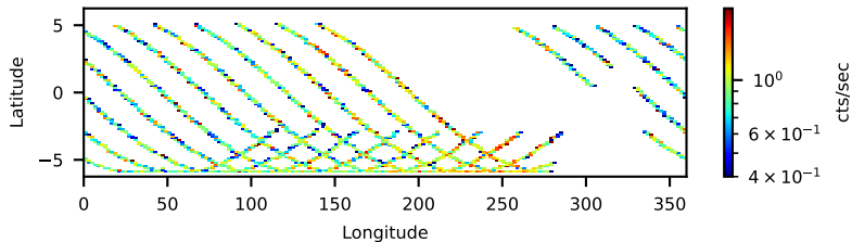
30460015002: 3 to 120 keV
