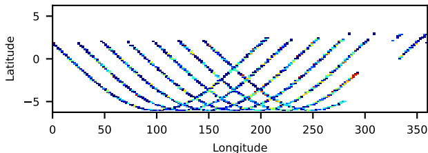
30402035002: 30 to 120 keV
