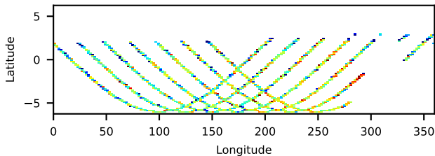
30402035002: 3 to 120 keV
