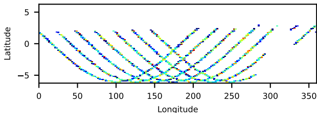
30402035002: 3 to 10 keV
