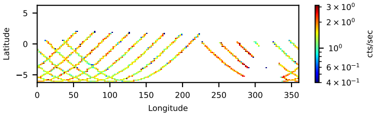
30363002002: 3 to 120 keV
