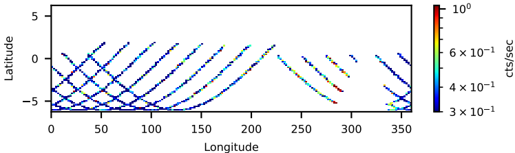
30363002002: 30 to 120 keV
