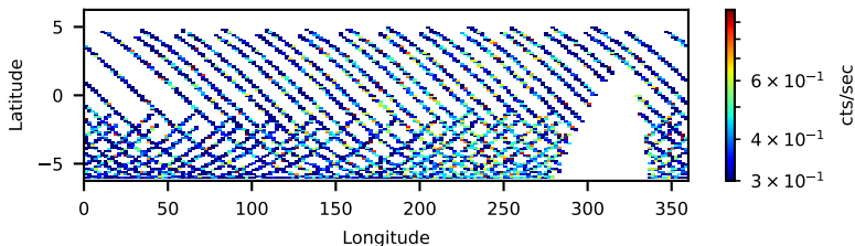
30361003002: 30 to 120 keV
