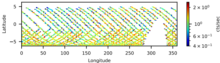
30361003002: 3 to 120 keV
