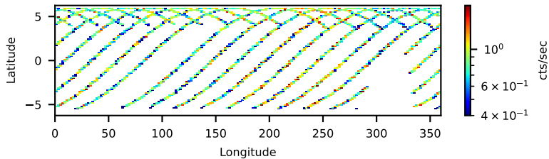
30360002002: 3 to 120 keV
