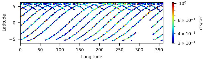
30360002002: 30 to 120 keV
