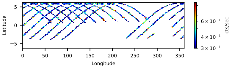
30301009002: 30 to 120 keV
