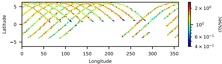
30301009002: 3 to 120 keV
