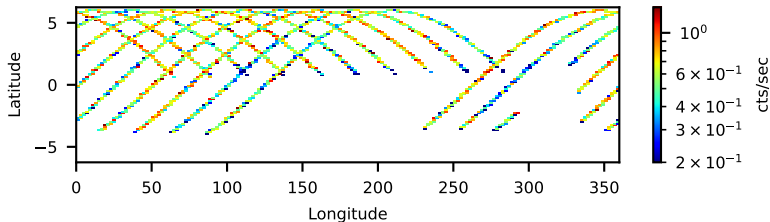
30301009002: 3 to 10 keV
