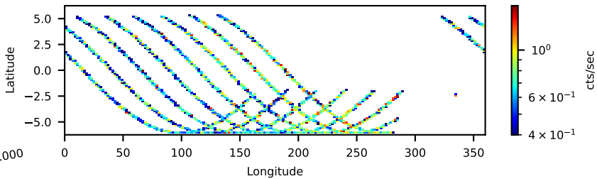
30202027008: 3 to 10 keV
