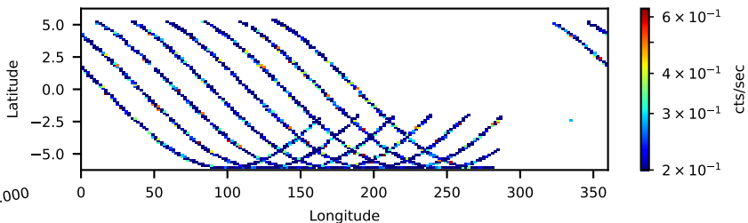
30202027008: 30 to 120 keV
