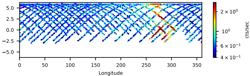
30101021002: 3 to 10 keV
