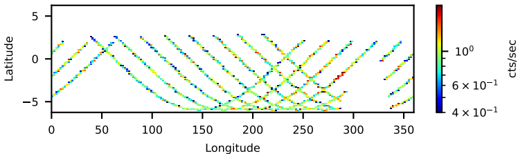
30101001002: 3 to 120 keV
