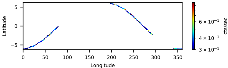
30002032001: 30 to 120 keV
