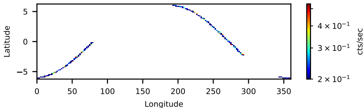
30002032001: 3 to 10 keV
