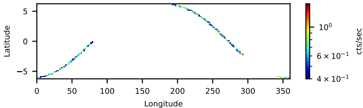
30002032001: 3 to 120 keV
