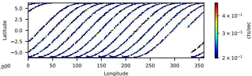
10802004002: 30 to 120 keV
