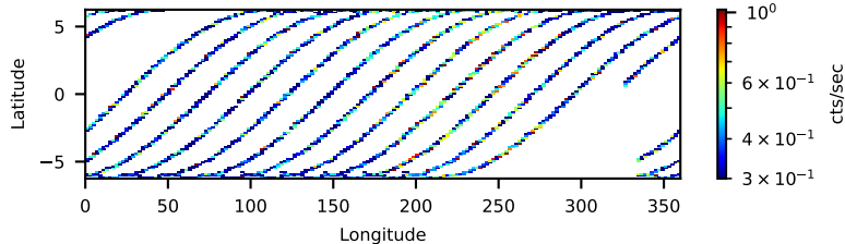
10802004002: 30 to 120 keV
