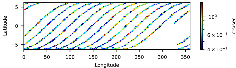
10802004002: 3 to 120 keV
