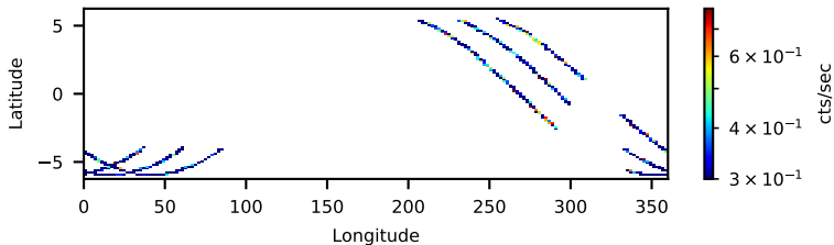
10702303004: 30 to 120 keV
