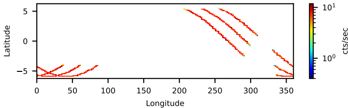
10702303004: 3 to 120 keV
