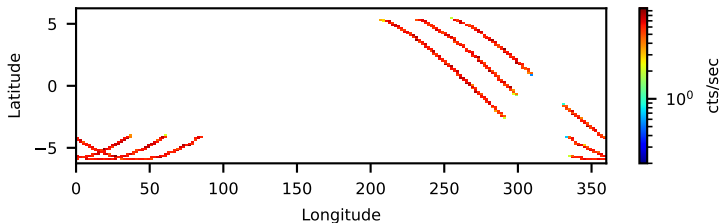
10702303004: 3 to 10 keV
