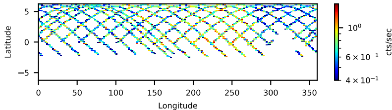
10602004002: 3 to 120 keV
