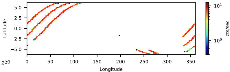
10602002008: 3 to 10 keV
