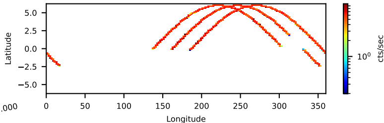
10602002004: 30 to 120 keV
