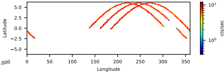
10602002004: 3 to 10 keV
