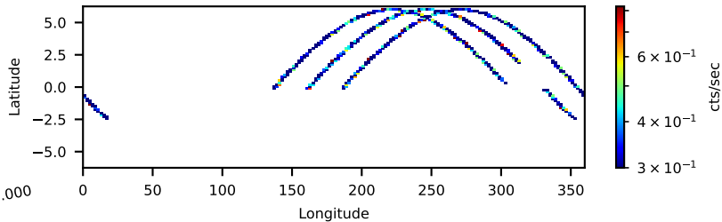
10602002004: 30 to 120 keV
