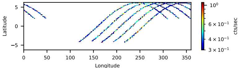
10502004004: 30 to 120 keV
