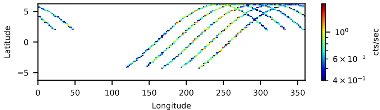
10502004004: 3 to 120 keV
