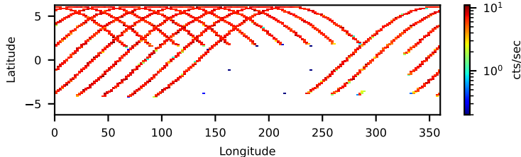
10502002004: 3 to 10 keV
