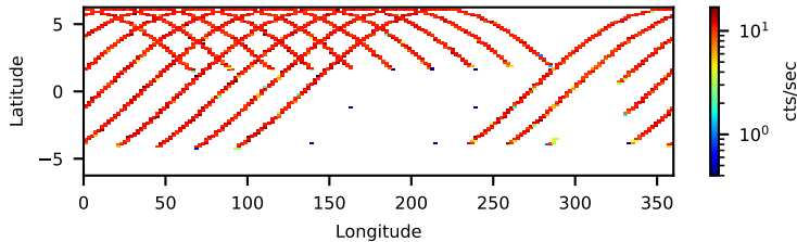
10502002004: 3 to 120 keV
