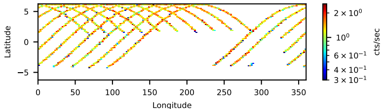
10502002004: 30 to 120 keV
